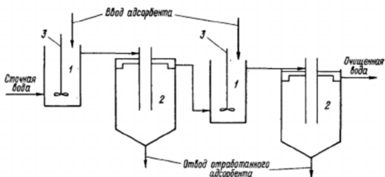
Рисунок 1. Схема адсорбционной установки в статических условиях: 1 – сорбционный реактор; 2 – отстойник; 3 – мешалка
