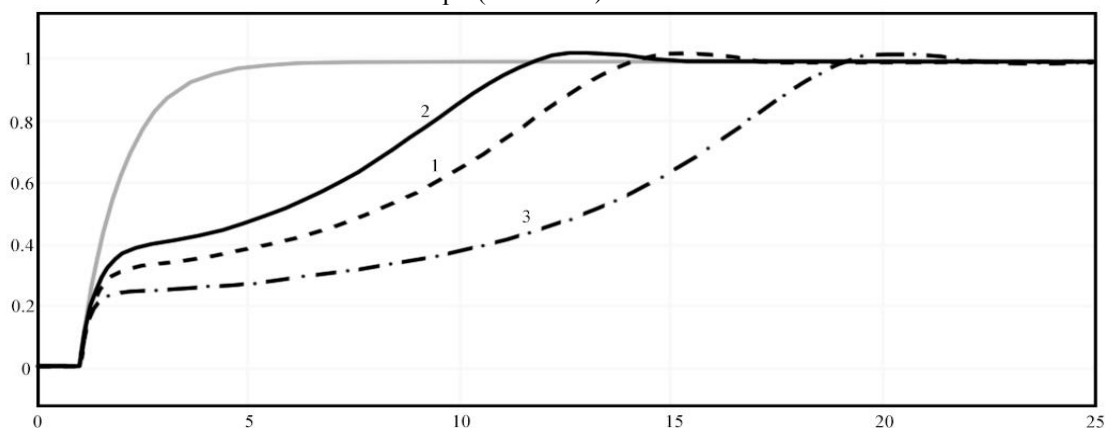
Рисунок 5 – График влияния параметра \lambda на быстродействие системы при действии сигнала step при a = 2 и (k_0 + a_0) = 1 : сплошная линия – требуемый сигнал; график 1 при \lambda = 1 ; график 2 при \lambda = 0,5 ; график 3 при \lambda = 2
