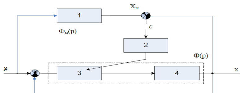
Рисунок 1 – Адаптивная система с эталонной моделью:
