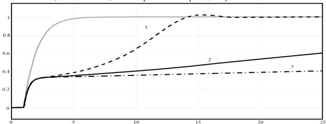
Рисунок 4 – График влияния параметра (k_0 + a_0) при действии сигнала step на выходной сигнал при a = 2 и \lambda = 1 : сплошная линия – требуемый сигнал; график 1 при (k_0 + a_0) = 1 ; график 2 при (k_0 + a_0) = 1,5 ; график 3 при (k_0 + a_0) = 2
