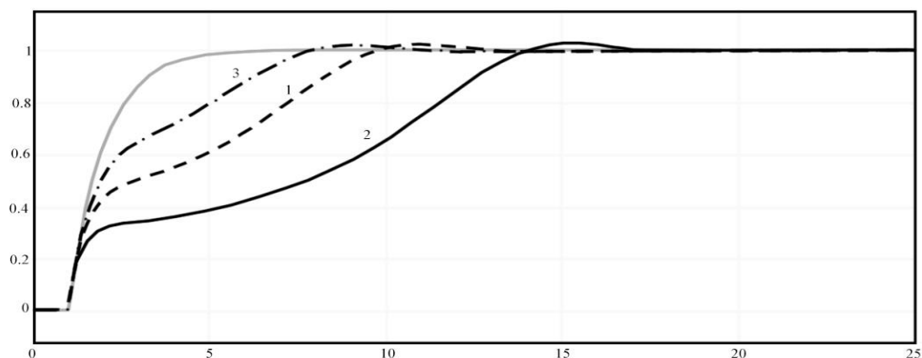
Рисунок 6 – График влияния параметра a на выходной сигнал при действии сигнала step : сплошная линия – требуемый сигнал; график 1 при a=1 ; график 2 при a=2 ; график 3 при a=0,5 при значениях ( k_0 + a_0 )=1 и \lambda=1
