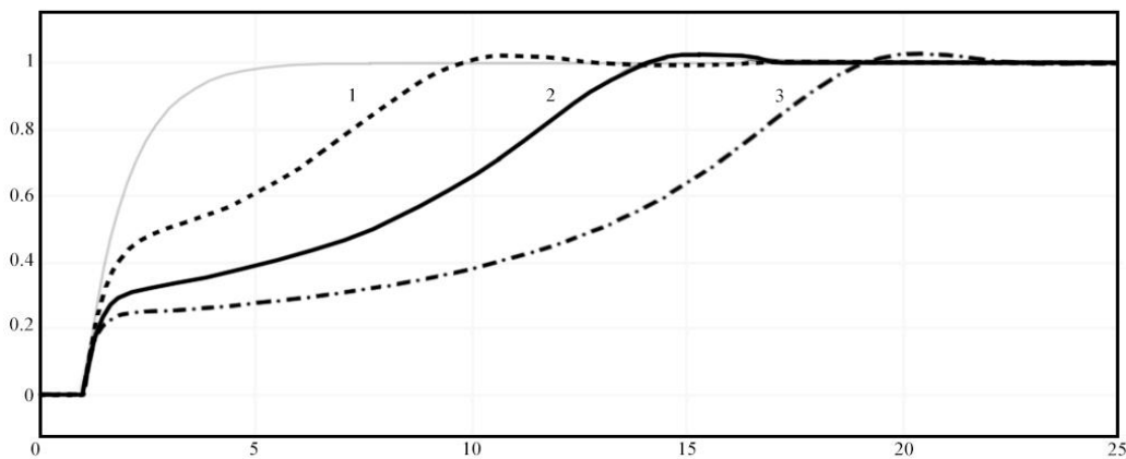
Рисунок 3 – Графики работы адаптивной системы при действии ступенчатого входного сигнала ( step ) и постоянных параметрах (k_0 + a_0) = 1 , \lambda = 1 : сплошная линия – требуемый сигнал; график 1 при ( a = 2 ); график 2 при ( a = 3 ); график 3 при ( a = 4 )
