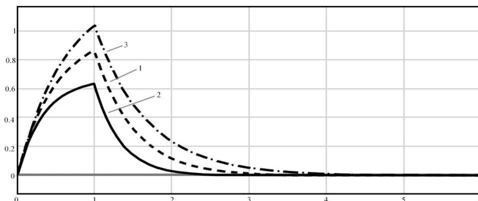
Рисунок 7 – График влияния параметра a на выходной сигнал при действии сигнала pulsegenerator : график 1 при a=1 ; график 2 при a=2 ; график 3 при a=0.5 ; (значения k_0 + a_0 = 1 и \lambda=1 постоянны)
