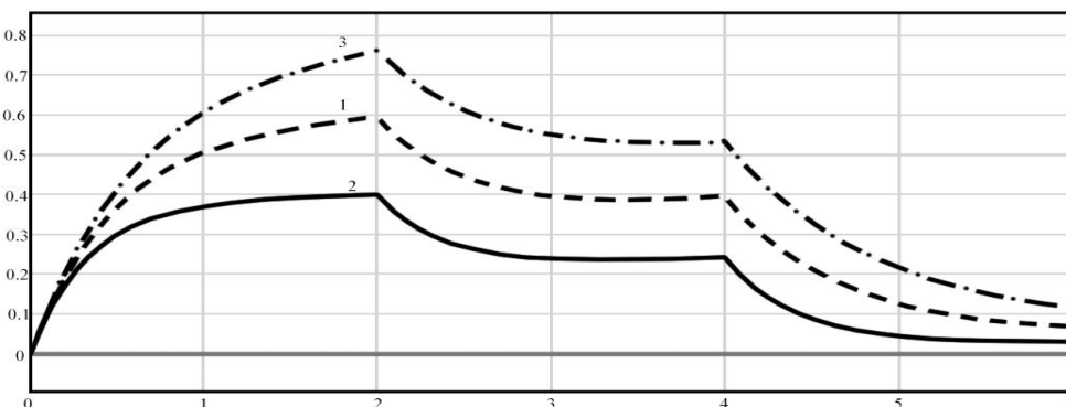
Рисунок 8 – График влияния параметра a на выходной сигнал при действии сигнала randomnumber : график 1 при a=1 ; график 2 при a=2 ; график 3 при a=0.5 ; (значения k_0 + a_0 = 1 , \lambda=1 постоянны)
