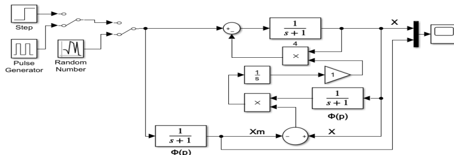
Рисунок 2 – Схема адаптивной системы с эталонной моделью в среде Matlab : X_m – выходная координата модели; X – входная координата модели; \Phi(p) – передаточная функция замкнутой системы
