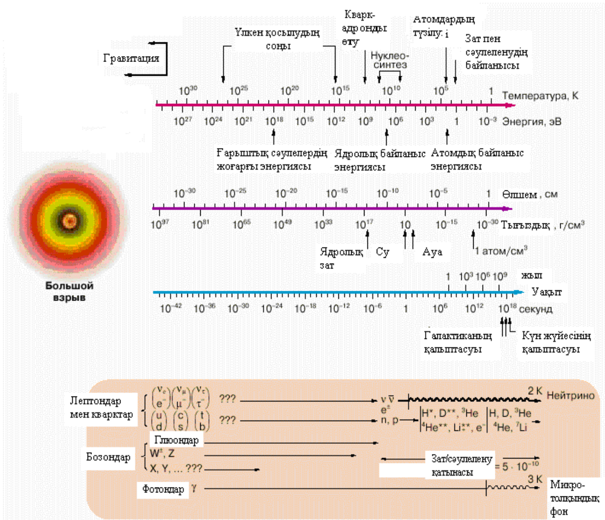
1-сурет. Ертедегі әлемдегі температураның, энергияның, уақыттың, өлшемнің, тығыздықтың байланысы. Схеманың төменгі бөлігі материяның кварктық және лептондық құрамын сипаттайды.
